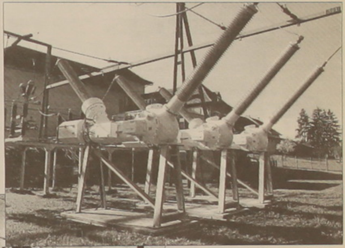
110 կՎ ենթակայանի վերազինումը ABB-ի ժամանակակից սարքավորումներով:
